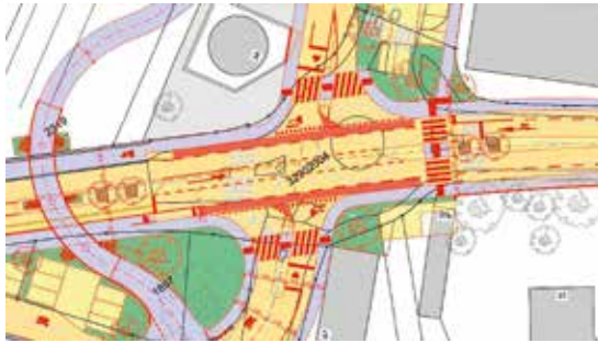
Plan des umgebauten Knotens Eisenbahn- strasse
